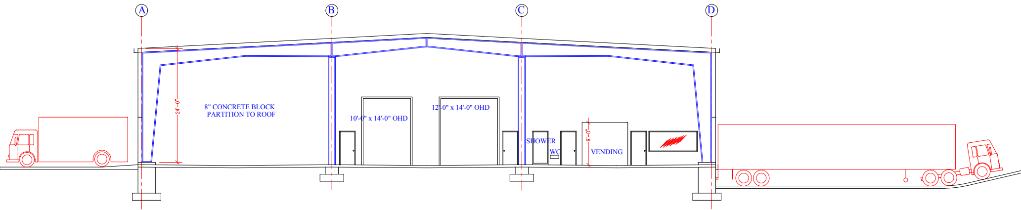
SECTION "B-B" SCALE: 1/8" = 1' - 0"
