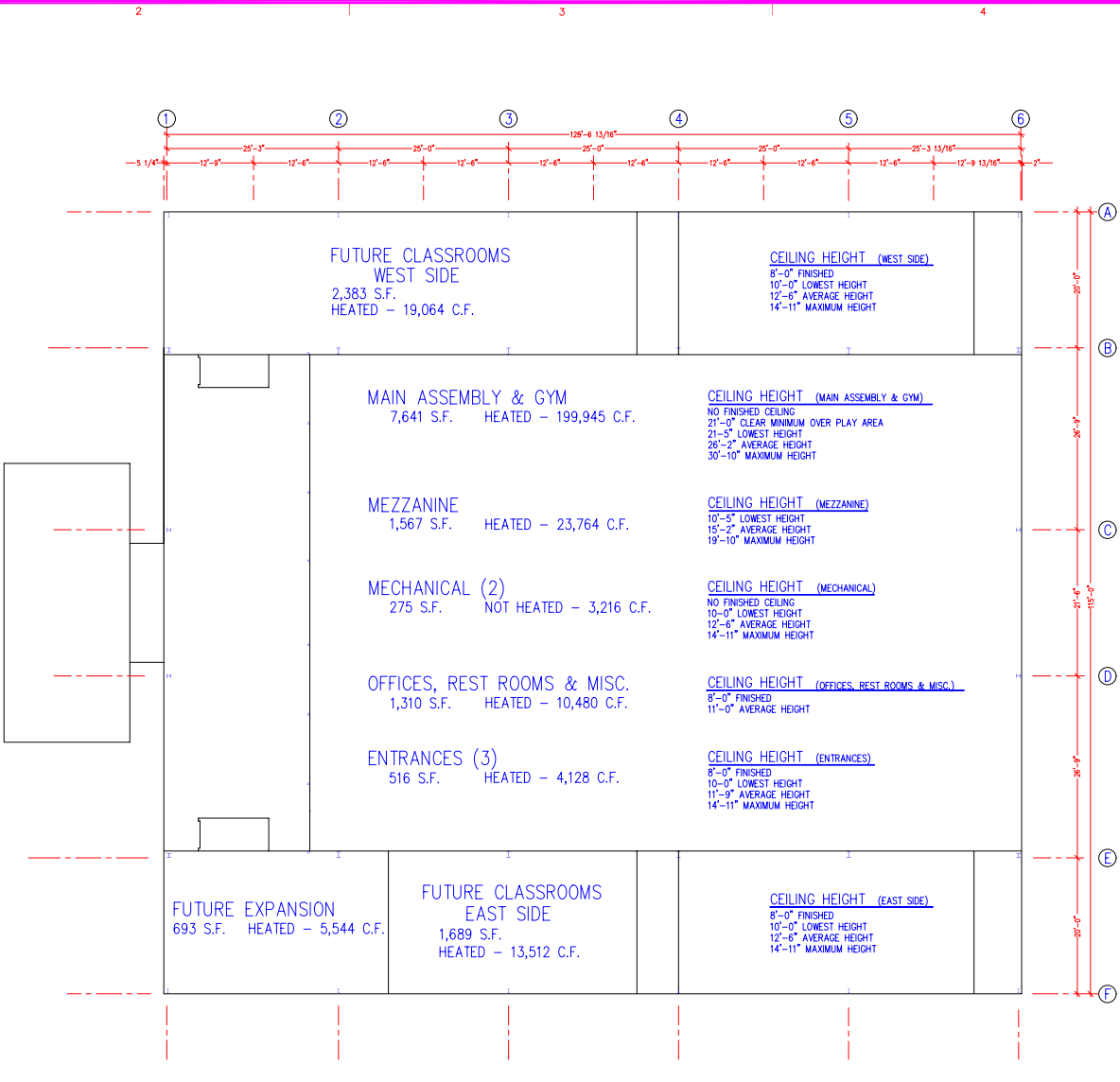
SCHMATIC PLAN SCALE: 1/8" = 1' - 0"
